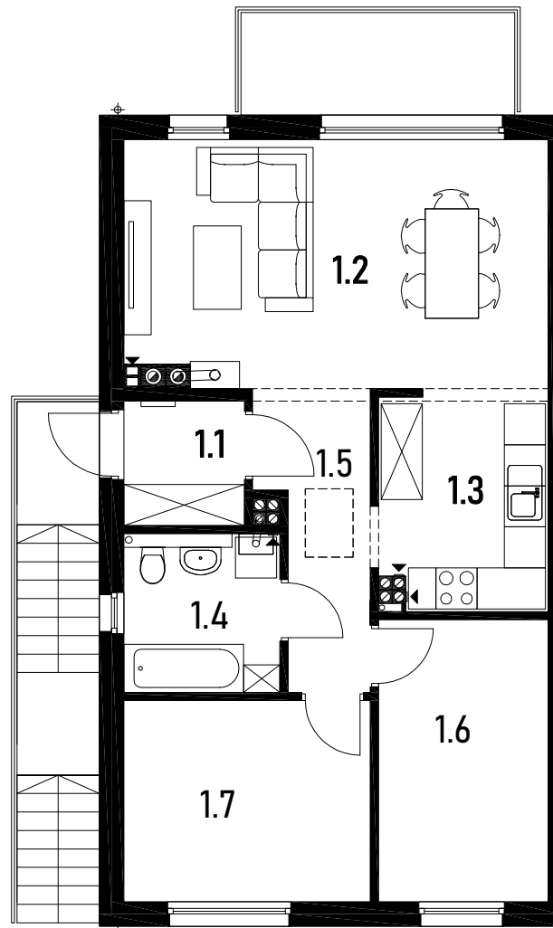
rzut kondygnacji 1:100
