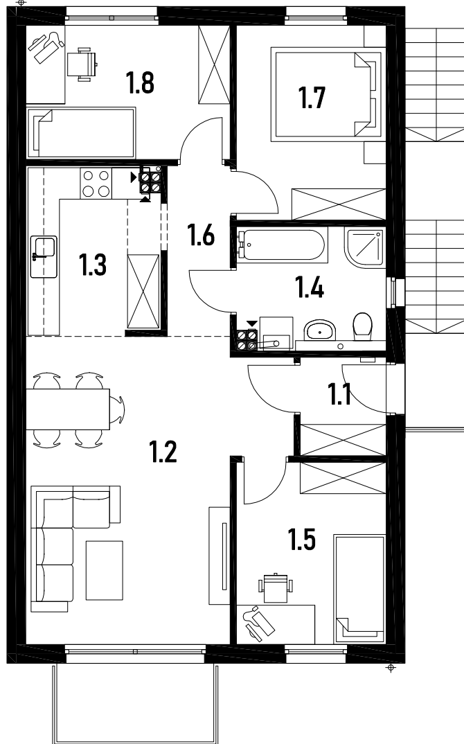
rzut kondygnacji 1:100
